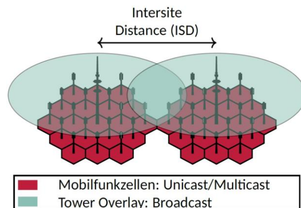
Abbildung 1: Ein Gleichwellennetz mit zwei Broadcast-Sendetürmen überlagert die klassischen Mobilfunkzellen. Der Abstand zwischen den Sendetürmen wird als Intersite-Distance (ISD) bezeichnet (alle Bilder: Jonas von Beöczy).
